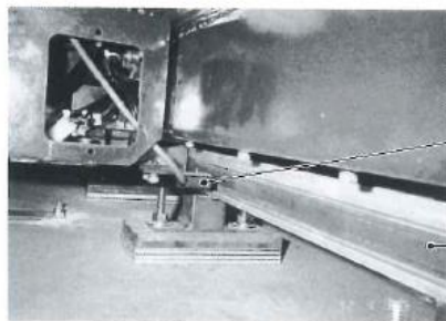
水平移動軸に取り付けられた MCスケールとヘッド
